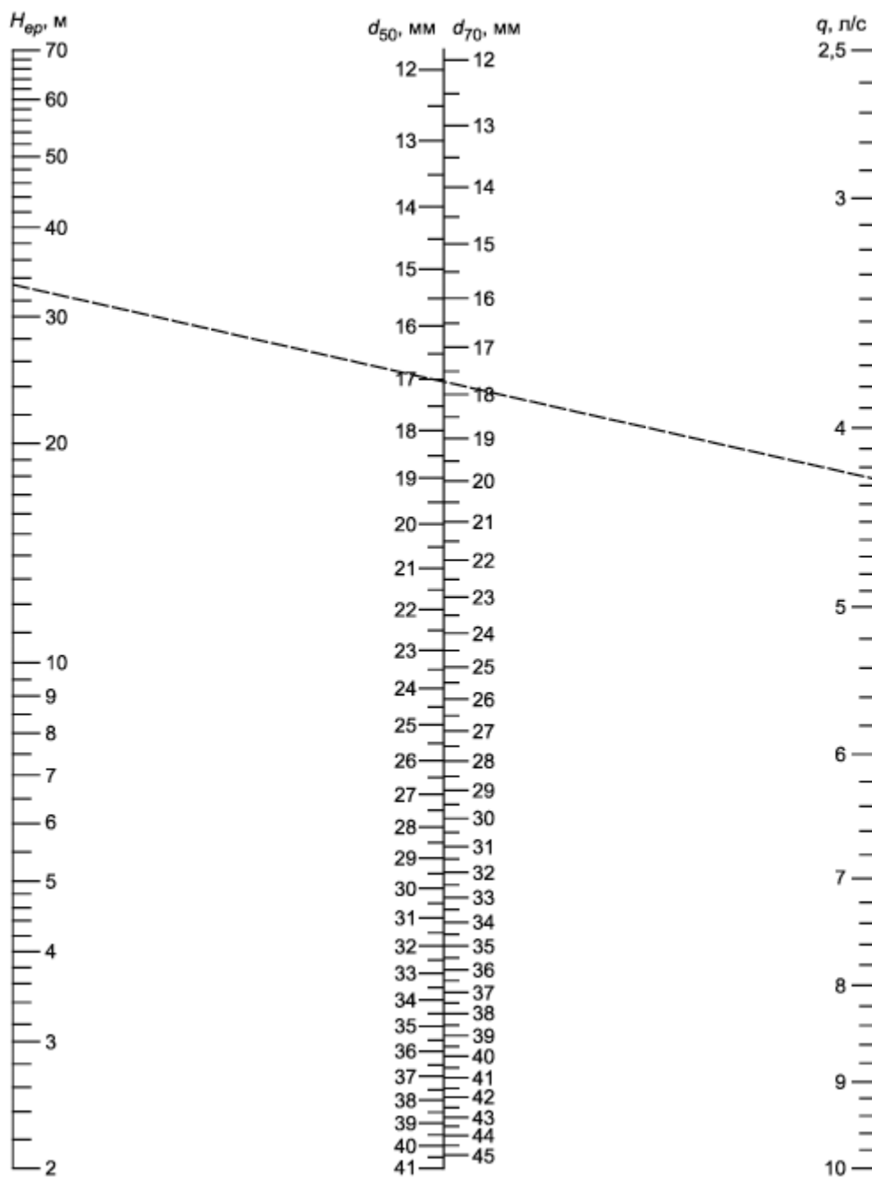
d_{50}, d_{70} - диаметры отверстий диафрагм, устанавливаемых у пожарных кранов диаметром 50, 65 (70) мм Рисунок В.1
